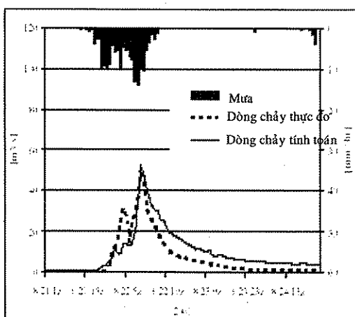
Hình 3. Dòng chảy đến đập Shimagawa (sử dụng số liệu mưa đo tại trạm khí tượng bề mặt)
