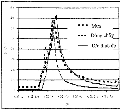
Hình 5. Đường quá trình lưu lượng thực đo và tính toán tại trạm Murakami. (sử dụng số liệu mưa đo tại trạm khí tượng bề mặt và số liệu mưa nội suy từ sản phẩm Radar)
