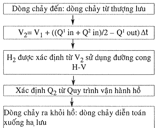
Hình 2. Sơ đồ mô hình vận hành hồ chứa
