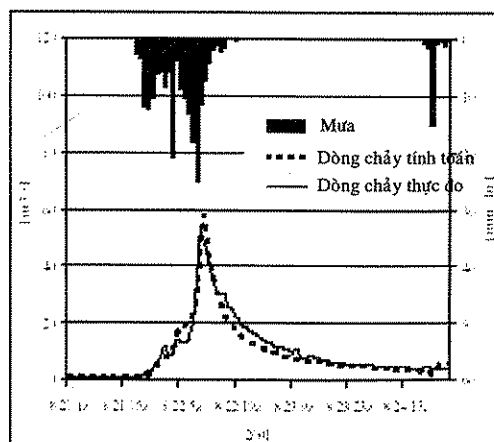
Hình 4. Dòng chảy đến đập Shimagawa (sử dụng số liệu mưa nội suy từ sản phẩm Radar)
