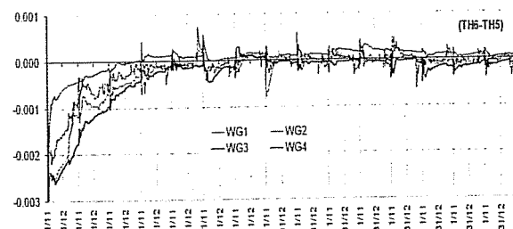
Hình 6. Biến thiên độ ẩm đất (WG) ở các lớp đất khác nhau trong 15 chu kỳ tích phân (TH4, TH5, TH6) và hiệu độ ẩm đất tương ứng giữa TH6 và TH4 (TH6-TH4), TH6 và TH5 (TH6-TH5). Trục tung là độ ẩm đất ( m^3/m^3 ), trục hoành là thời gian. Các chỉ số sau WG tương ứng với các lớp đất: 1 (0-10cm), 2 (10-40cm), 3 (40-100cm) và 4 (100-200cm)
