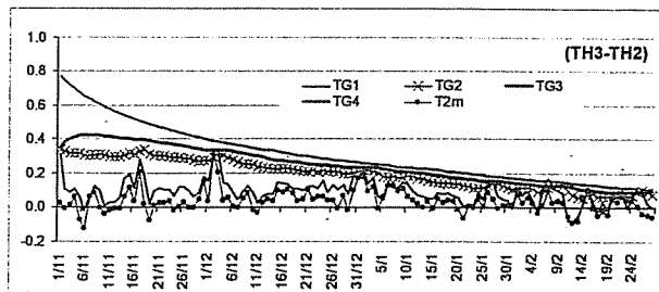
Hình 1. Biến thiên nhiệt độ không khí ( T_{2m} ) và nhiệt độ đất (TG) ở các lớp đất khác nhau trong một chu kỳ tích phân (TH1, TH2, TH3) và hiệu nhiệt độ tương ứng giữa TH3 và TH1 (TH3-TH1), TH3 và TH2 (TH3-TH2). Trục tung là nhiệt độ ( ^{\circ}\text{C} ), trục hoành là thời gian. Các chỉ số sau TG tương ứng với các lớp đất: 1 (0-10cm), 2 (10-40cm), 3 (40-100cm) và 4 (100-200cm)
