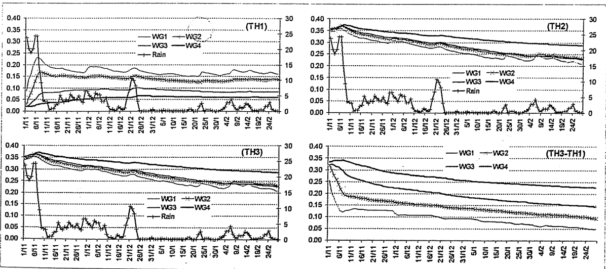
Hình 2. Biến thiên lượng mưa ngày và độ ẩm đất (WG) ở các lớp đất khác nhau trong một chu kỳ tích phân (TH1, TH2, TH3) và hiệu độ ẩm đất tương ứng giữa TH3 và TH1 (TH3-TH1), TH3 và TH2 (TH3-TH2). Trục tung là độ ẩm đất ( \text{m}^3/\text{m}^3 ), trục hoành là thời gian. Các chỉ số sau WG tương ứng với các lớp đất: 1 (0-10cm), 2 (10-40cm), 3 (40-100cm) và 4 (100-200cm)
