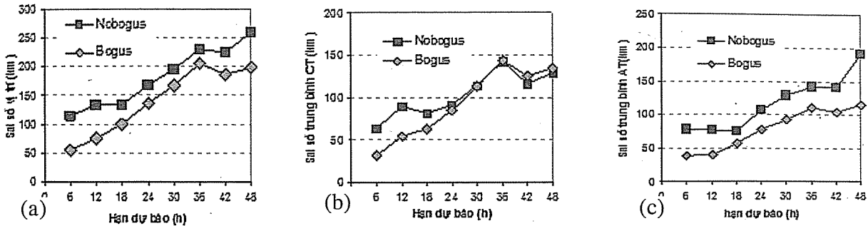
Hình 3. Sai số vị trí trung bình MPE (a), sai số CT trung bình (b) và sai số AT trung bình (c) của các trường hợp dự báo thử nghiệm.
