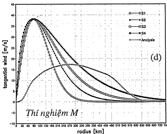
Hình 1. Profile gió tiếp tuyến theo bán kính trong các thí nghiệm RM, S, M và hàm trọng số theo áp suất của thí nghiệm W. Các hình minh họa sử dụng trường hợp bão Imbudo 12h 22/7/2003
