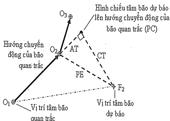
Hình 2. Sơ đồ mô tả cách xác định sai số tốc độ (AT) và hướng (CT) của quỹ đạo dự báo. PE là sai số vị trí; O_1, O_2, O_3 là các vị trí tâm bão quan trắc; F_2 là vị trí tâm bão dự báo ứng với vị trí tâm quan trắc O_2
