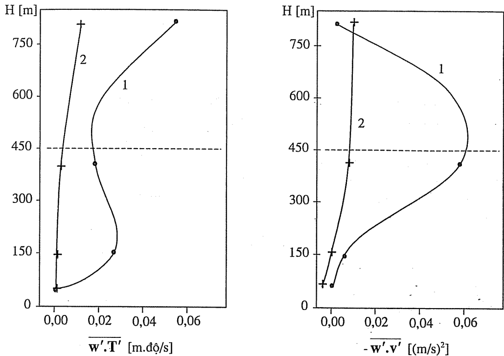
Hình 3. Profin thẳng đứng của các dòng rối toàn phần của nhiệt độ và động lượng trong lớp biên (1) và profin tương ứng của các dòng rối tính đến mạch động quy mô nhỏ ( \lambda < 500 \text{ m} ), nhận được nhờ lọc tuyến tính (2).
