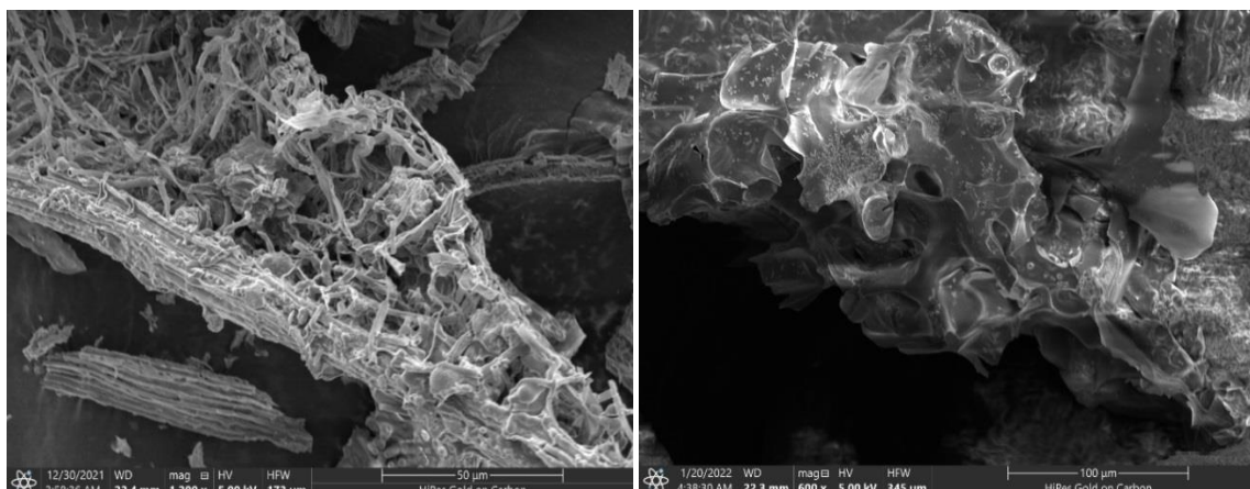
Hình 3. Ảnh SEM bề mặt than sinh học trước ( \times 1200 mag.) và sau hấp phụ ( \times 600 mag.).
