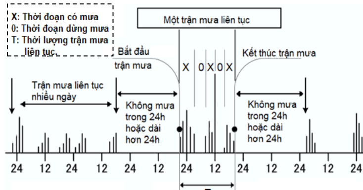
Hình 2. Minh họa định nghĩa và cách tính thời lượng một trận mưa liên tục [15].
