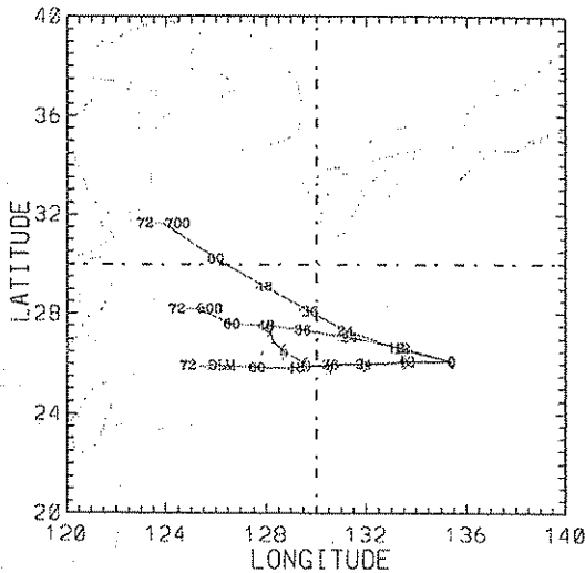
c) JELEWAT
