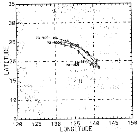
b) SAOMAI
