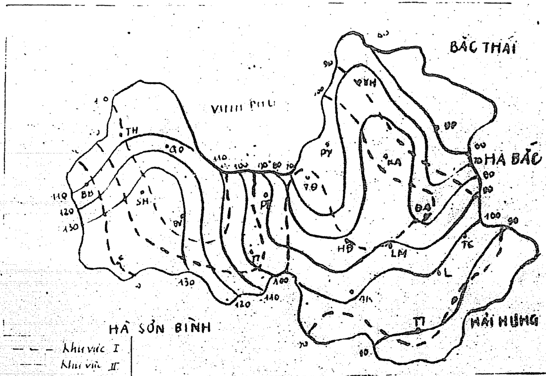
Bản đồ 3. Lượng mưa trung bình 3 ngày y khi bão vào khu vực I và II
