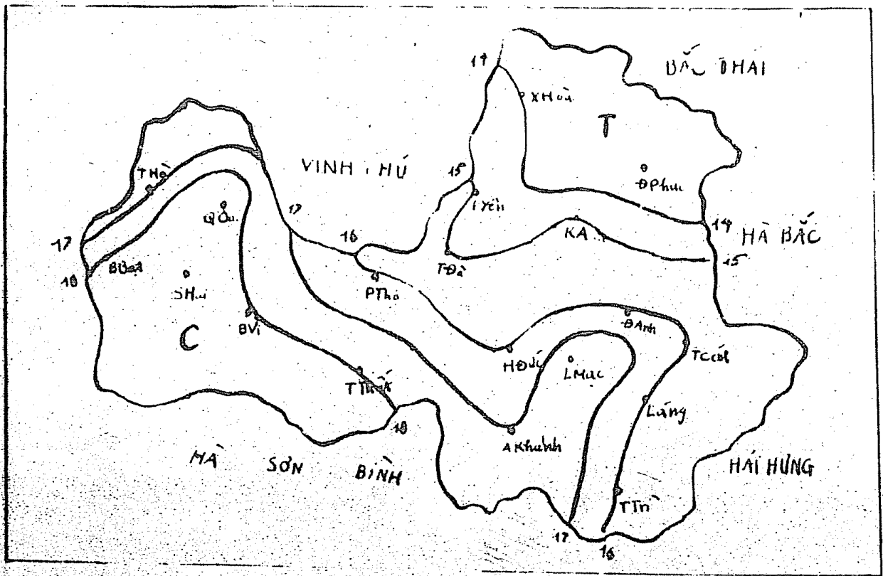
B ả n đồ 1. Phân bố tỷ trọng mưa b ̄ao ở Hà Nội
