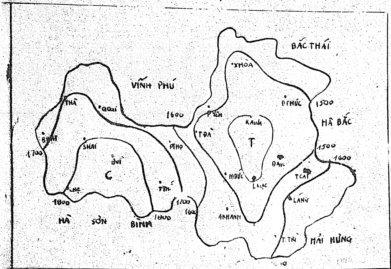
B ả n đồ 2. Phân bố lượng mưa năm TBNN ở Hà Nội
