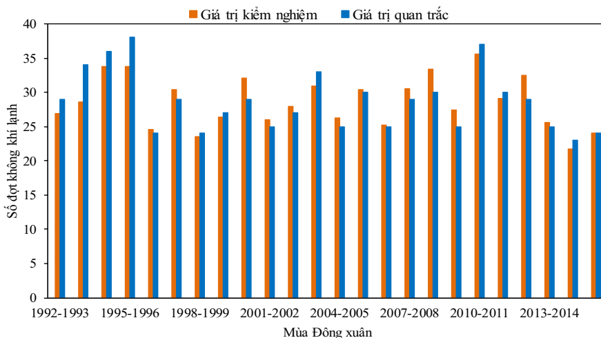
Hình 2. Tương tự như hình 1 nhưng cho phương trình dự báo dựa trên 4 chỉ số I_{LiYang} , I_{Jhun} , I_{Yang} và I_{SUN}
