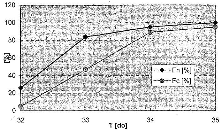
Hình 4. Suất bảo đảm nhiệt độ nước Trạm Côn Đảo (1980-1998)
