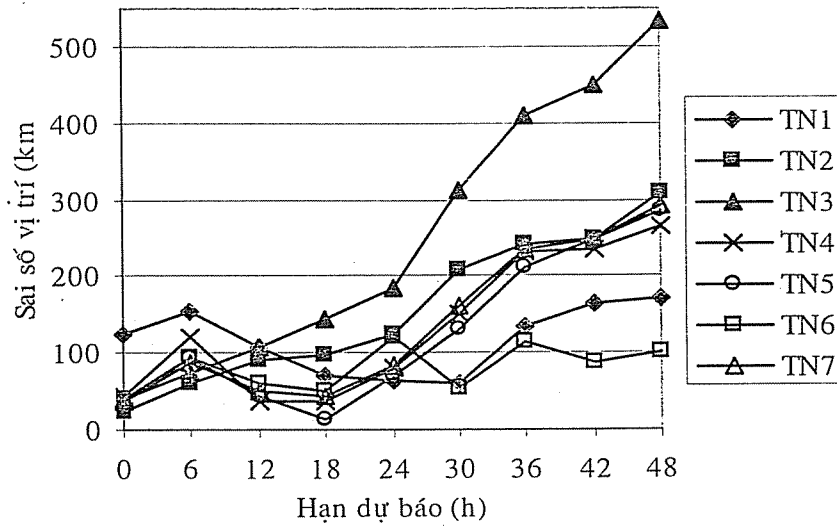
Hình 4. Quỹ đạo dự báo theo các trường hợp TN1-TN7 (đánh số từ 1-7) và quỹ đạo thực (hình xoáy bão) cơn bão NEPARTAK, 00UTC ngày 16/XI/2003 (D14) (a); và sai số vị trí theo các hạn dự báo (b)
