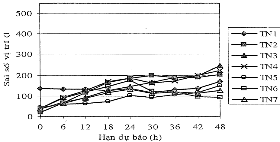
Hình 6. Sai số vị trí trung bình 4 trường hợp dự báo
