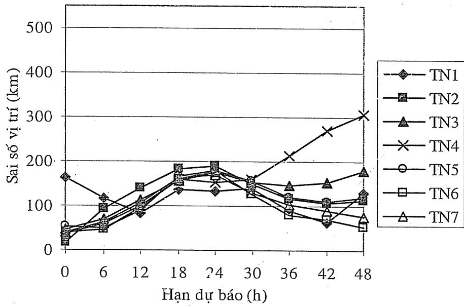
Hình 5. Quỹ đạo dự báo theo các trường hợp TN1-TN7 (đánh số từ 1-7) và quỹ đạo thực (hình xoáy bão) cơn bão NEPARTAK, 00UTC ngày 14/XI/2003 (D14) (a); và sai số vị trí theo các hạn dự báo (b)
