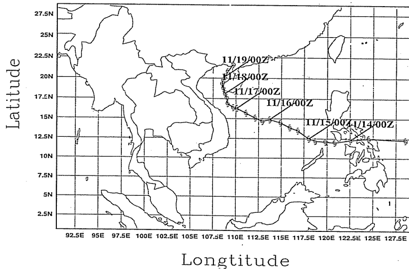
Hình 1. Đường đi cơn bão NEPARTAK (13-19/XI/2003; nguồn: weather.unisys.com) và miền dự báo của mô hình MM5.
