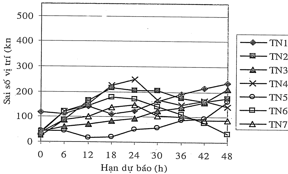
Hình 3. Quỹ đạo dự báo theo các trường hợp TN1-TN7 (đánh số từ 1-7) và quỹ đạo thực (hình xoáy bão) cơn bão NEPARTAK, 00UTC ngày 15/XI/2003 (D14) (a); và sai số vị trí theo các hạn dự báo (b)
