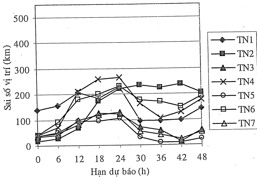
Hình 2. Quỹ đạo dự báo theo các trường hợp TN1- TN7 (đánh số từ 1-7) và quỹ đạo thực (hình xoáy bão) cơn bão NEPARTAK, 00UTC ngày 14/XI/2003 (D14) (a); và sai số vị trí theo các hạn dự báo (b)
