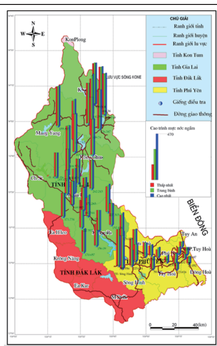
Hình 3. Mực nước ngầm tại các vị trí điều tra trên lưu vực sông Ba
