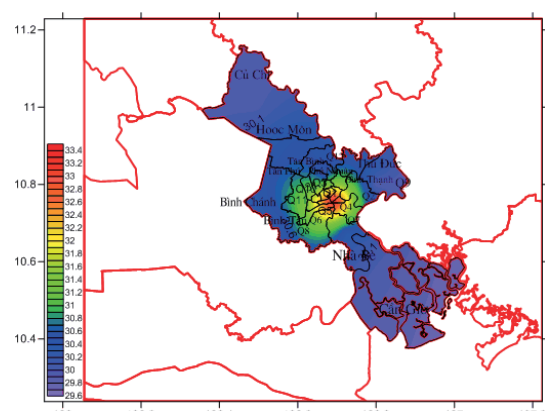
Hình 10. Nhiệt độ bề mặt trung bình tại TPHCM từ 01/08-15/08/2015
