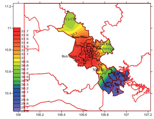
Hình 8. Nhiệt độ bề mặt tại TPHCM ngày 01/08/2015
