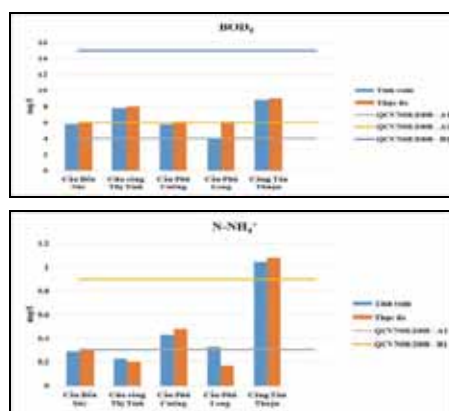
Hình 7. Kết quả tính toán hiệu chỉnh nồng độ các chất với số liệu thực đo các trạm dọc sông Sài Gòn tháng 7 năm 2014
