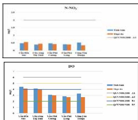
Hình 7. Kết quả tính toán hiệu chỉnh nồng độ các chất với số liệu thực đo các trạm dọc sông Sài Gòn tháng 7 năm 2014
