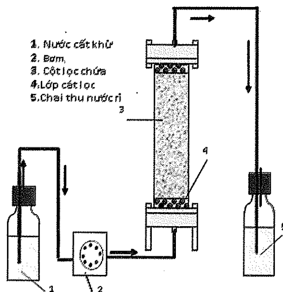
Hình 1. Sơ đồ thí nghiệm và mô hình xây dựng trong phòng thí nghiệm [DIN E 19528 (2007)]
