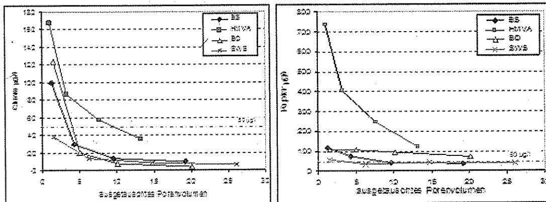
Hình 3. Biến thiên nồng độ kim loại chrom (trái) và đồng (phải) trong nước rỉ rác từ chất thải nghiên cứu (giá trị nồng độ cho phép 50 \mu\text{g/l} )
