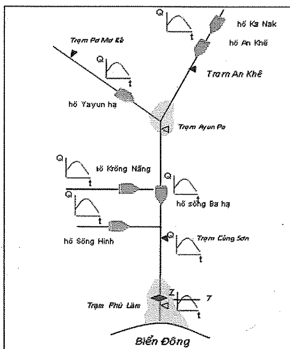
Hình 1. Sơ đồ hệ thống hồ chứa lớn trên sông Ba
