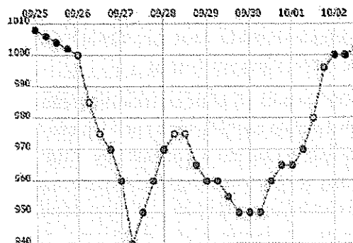
Hình 3. Áp suất trung bình của bão
