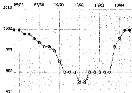
Hình 6. Biểu đồ áp suất trung bình của bão
