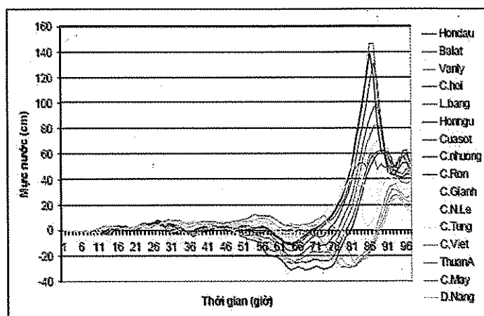
Hình 7. Mức nước dâng tại các trạm ven biển VN khi có bão Lekima
