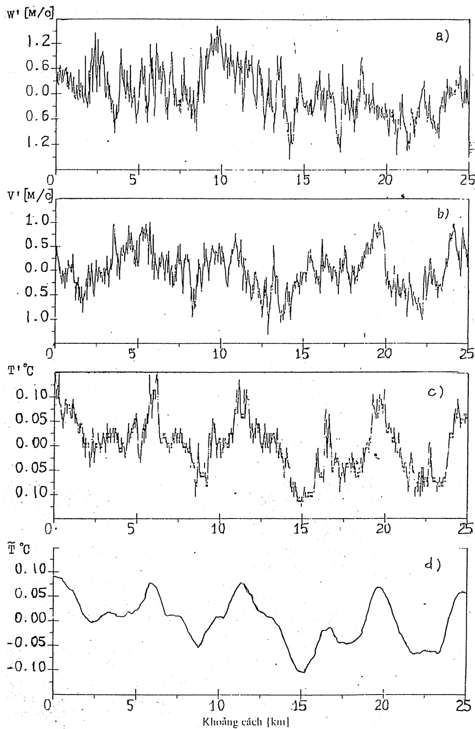
Hình 2. Mạch động, tương ứng với các thành phần thẳng đứng (a), nằm ngang (b) của tốc độ gió và nhiệt độ (c) và nhiệt độ qua bộ lọc (d) ở độ cao 170 m.
