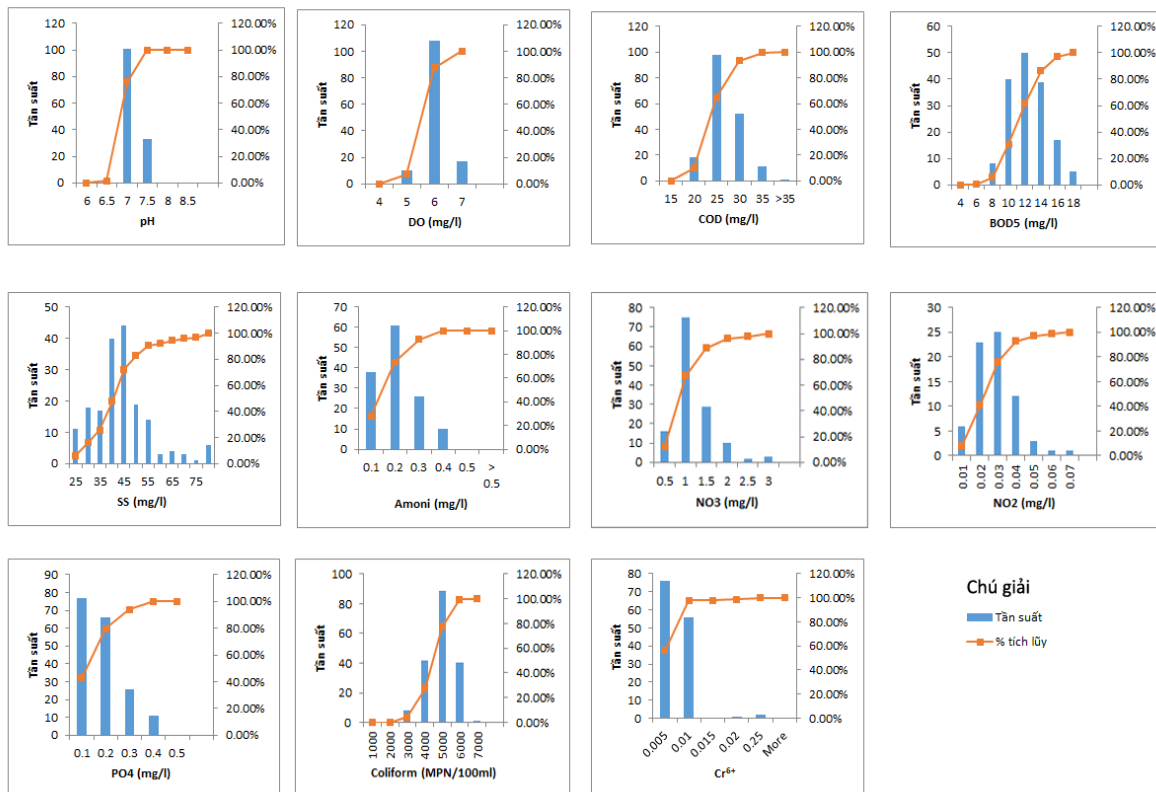
Hình 2. Phân bố nồng độ các chất ô nhiễm giai đoạn 2011–2019.
