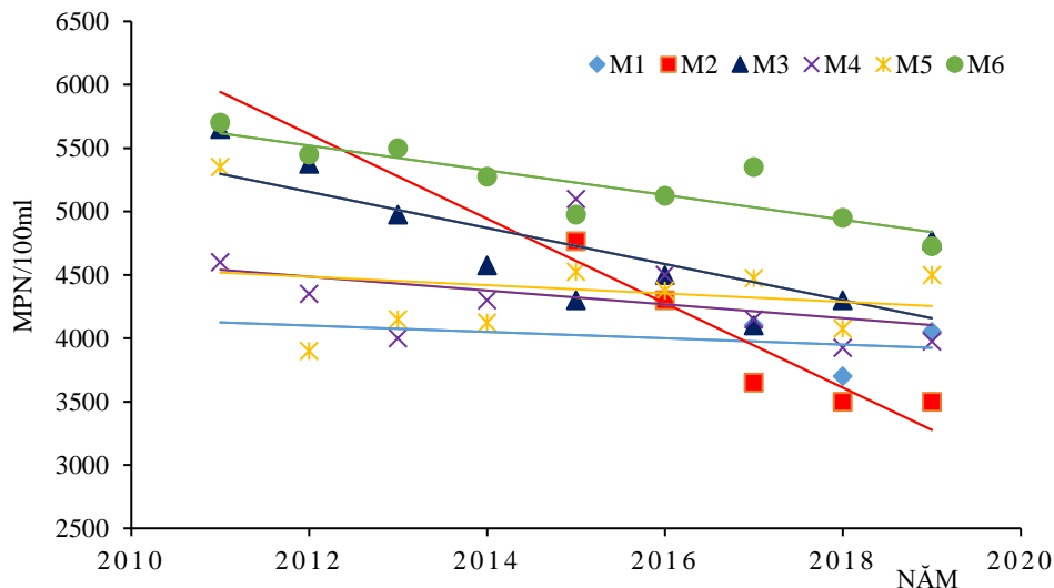
Hình 9. Diễn biến Coliform giai đoạn 2011–2019.
