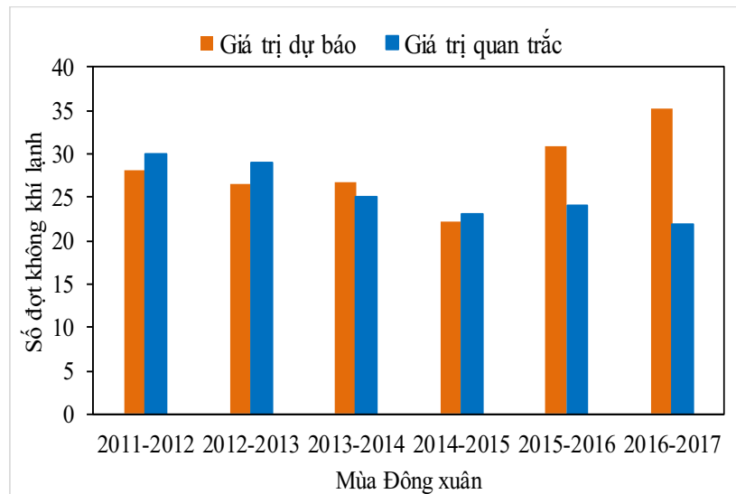
Hình 3. Số đợt KKL quan trắc được trong các tháng chính đông (màu xanh dương) và số đợt KKL dự báo tương ứng (màu cam) từ phương trình dự báo sử dụng 4 chỉ số I_{LiYang} , I_{Jhun} , I_{Yang} và I_{SUN} trong giai đoạn 2011-2016 sử dụng số liệu dự báo hạn mùa bắt đầu từ tháng 8 của ECMWF
