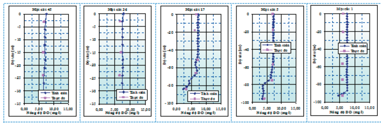
Hình 8. DO tính toán và thực đo tại các mặt cắt kiểm tra tháng 12 năm 2004
