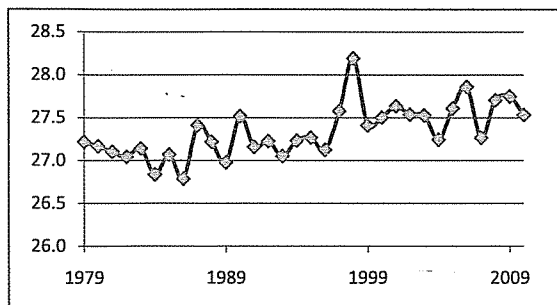
Hình 2. Biểu trình nhiệt độ trung bình năm tại Vũng Tàu giai đoạn 1979-2010
