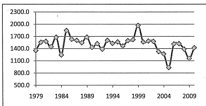
Hình 1. Biểu trình lượng mưa năm tại Vũng Tàu giai đoạn 1979-2010
