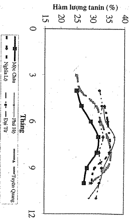
Hình 2. Động thái hàm lượng tannin chứa trong búp chè Trung du ở các vùng trồng chè khác nhau
