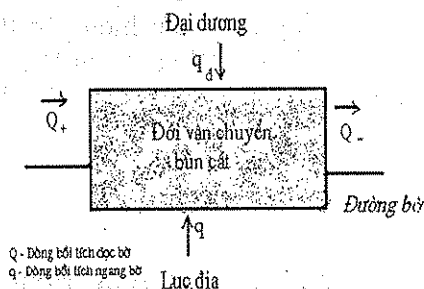
Hình 1. Cân bằng bùn cát trong khu bờ
