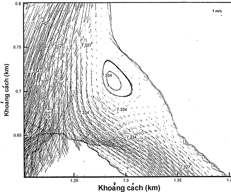
Hình 5 - Trường hợp mực nước +7,2 m - Mỏ cống Xuân Quan (Khu vật đầu cửa lấy nước)
