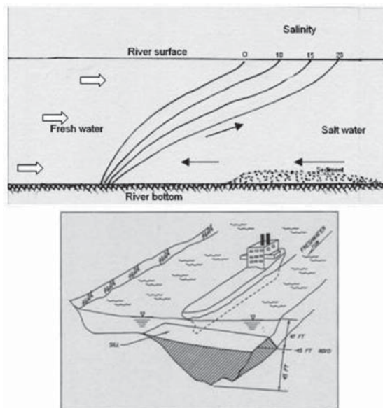
Hình 2. Tiết diện lưới nước mặn và hình dạng đập ngầm
